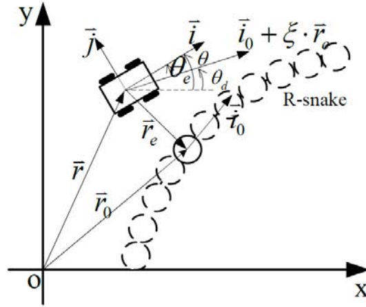
Fig. 3. Coordinates definitions
