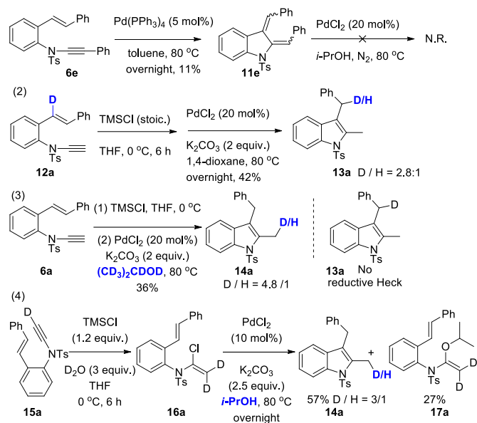
Scheme 3. Deuterium labelling study
